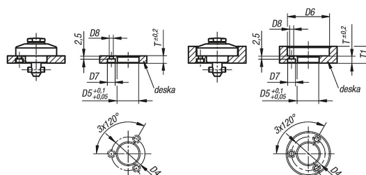
Možnost montáže, tvar A
