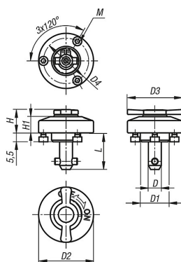
Možnost montáže, tvar B
